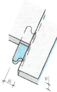
Detail "Schwalbenschwanz"
